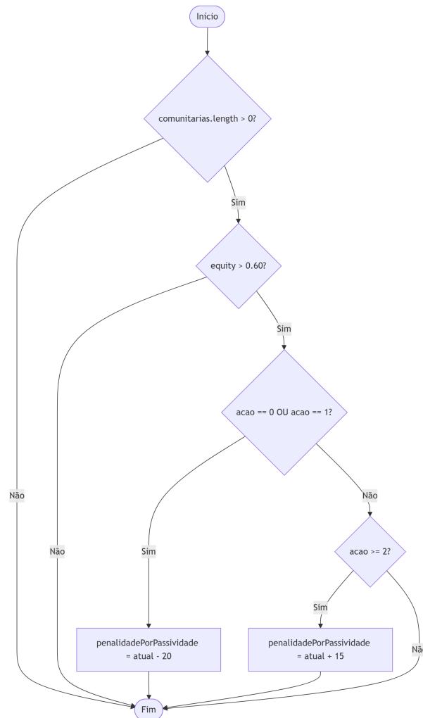
Figura 2 – Fluxograma do sistema de penalidade por passividade: Autoria própria
