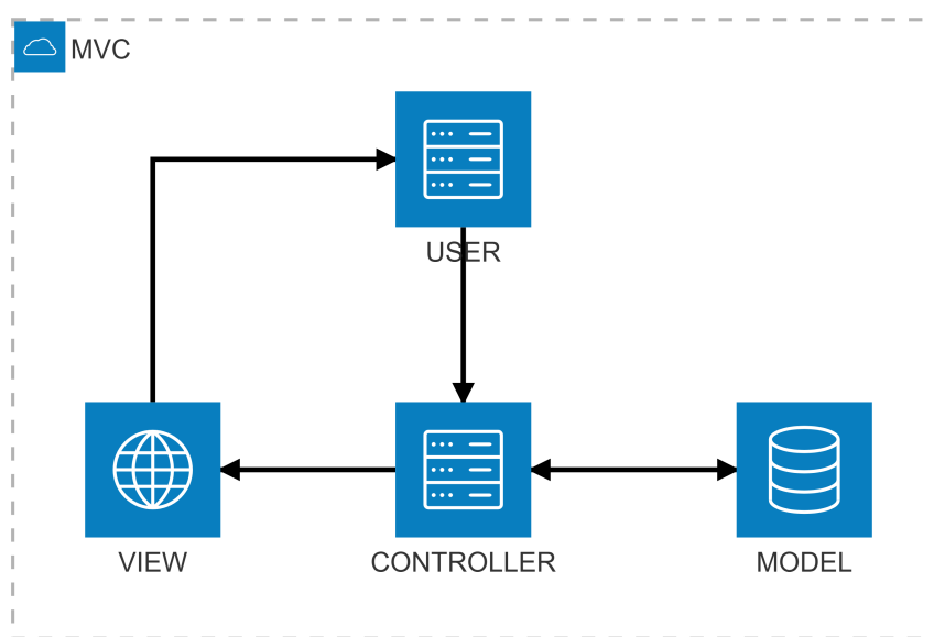
Figura 1 – Arquitetura MVC: Autoria própria
